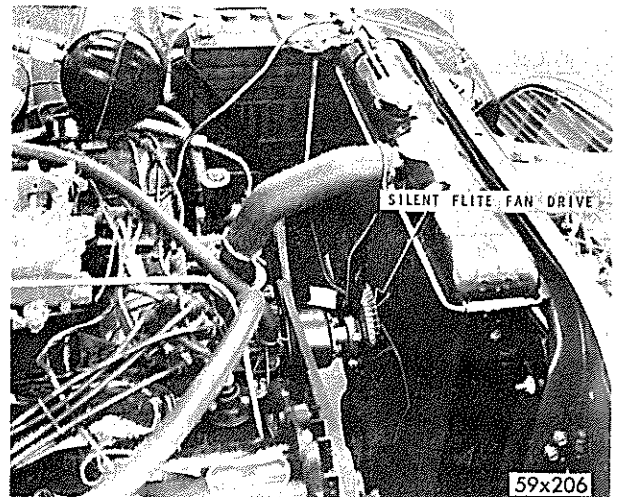
Fig. 2 - Silent Flite Fan Drive
